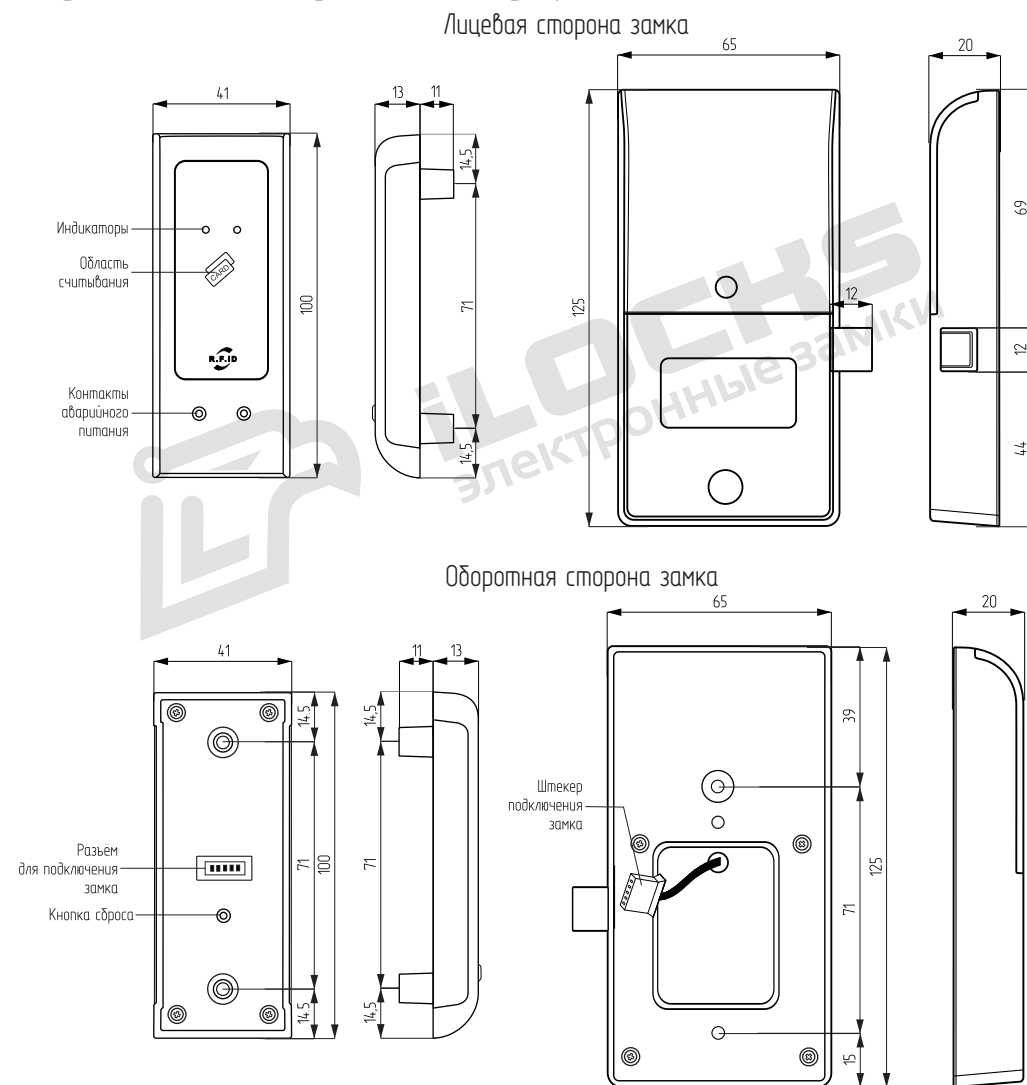
Рисунок №1 – Габаритные характеристики электронного замка для шкафчиков IS0600-MF
