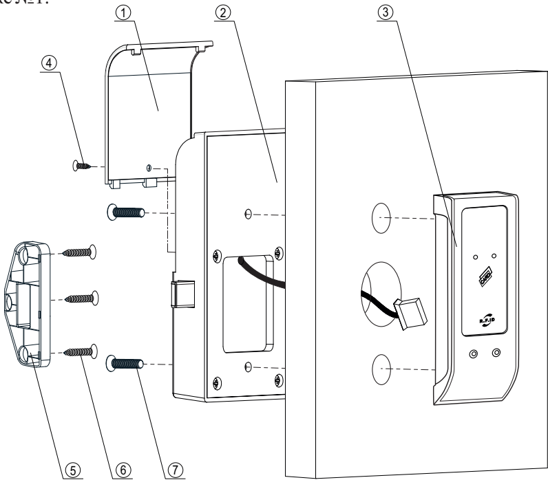
Рисунок №2 – Структурная схема (спецификация) электронного замка для шкафчиков IS0600-MF
