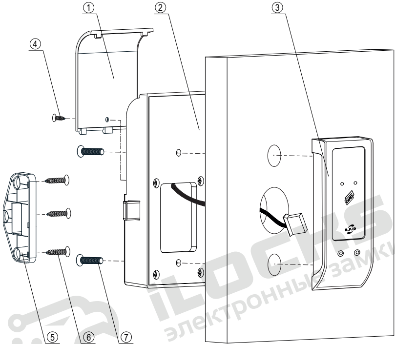
Рисунок №1 – Структурная схема (спецификация) электронного замка для шкафчиков IS0600-MF
