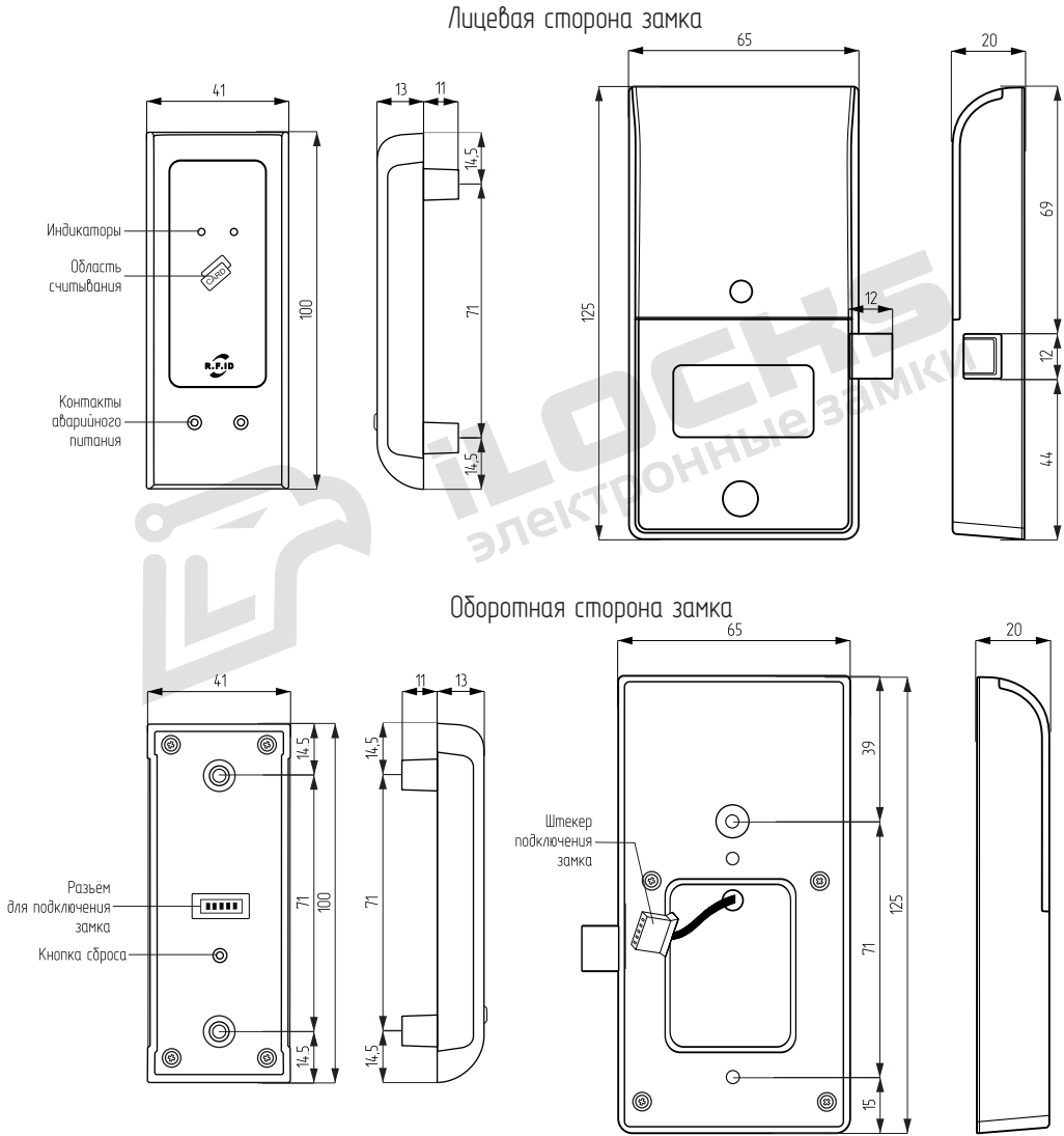
Рисунок №2 – Габаритные характеристики электронного замка для шкафчиков IS0600-MF
