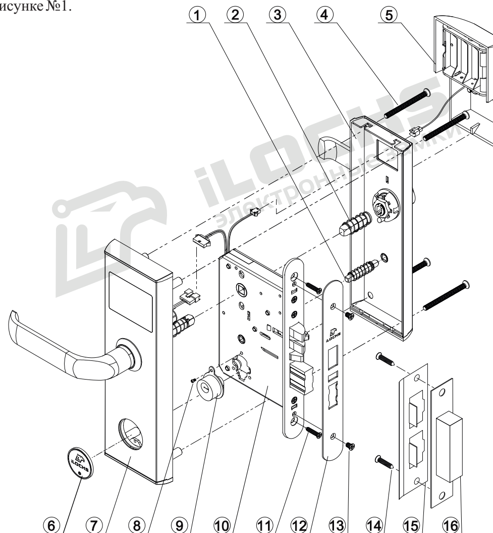
Рисунок №1 – Структурная схема (спецификация) замков типа iLOCKS IS8005A3B3
